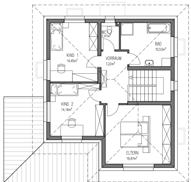
Obergeschoss
