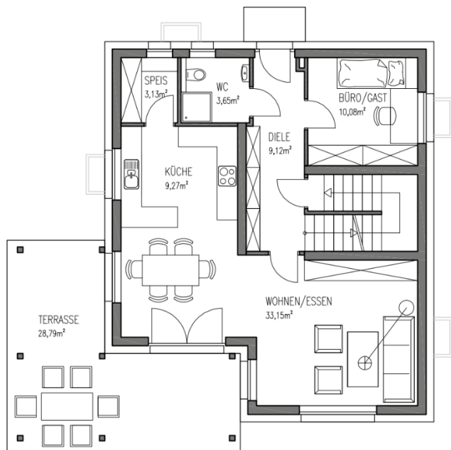
Erdgeschoss
